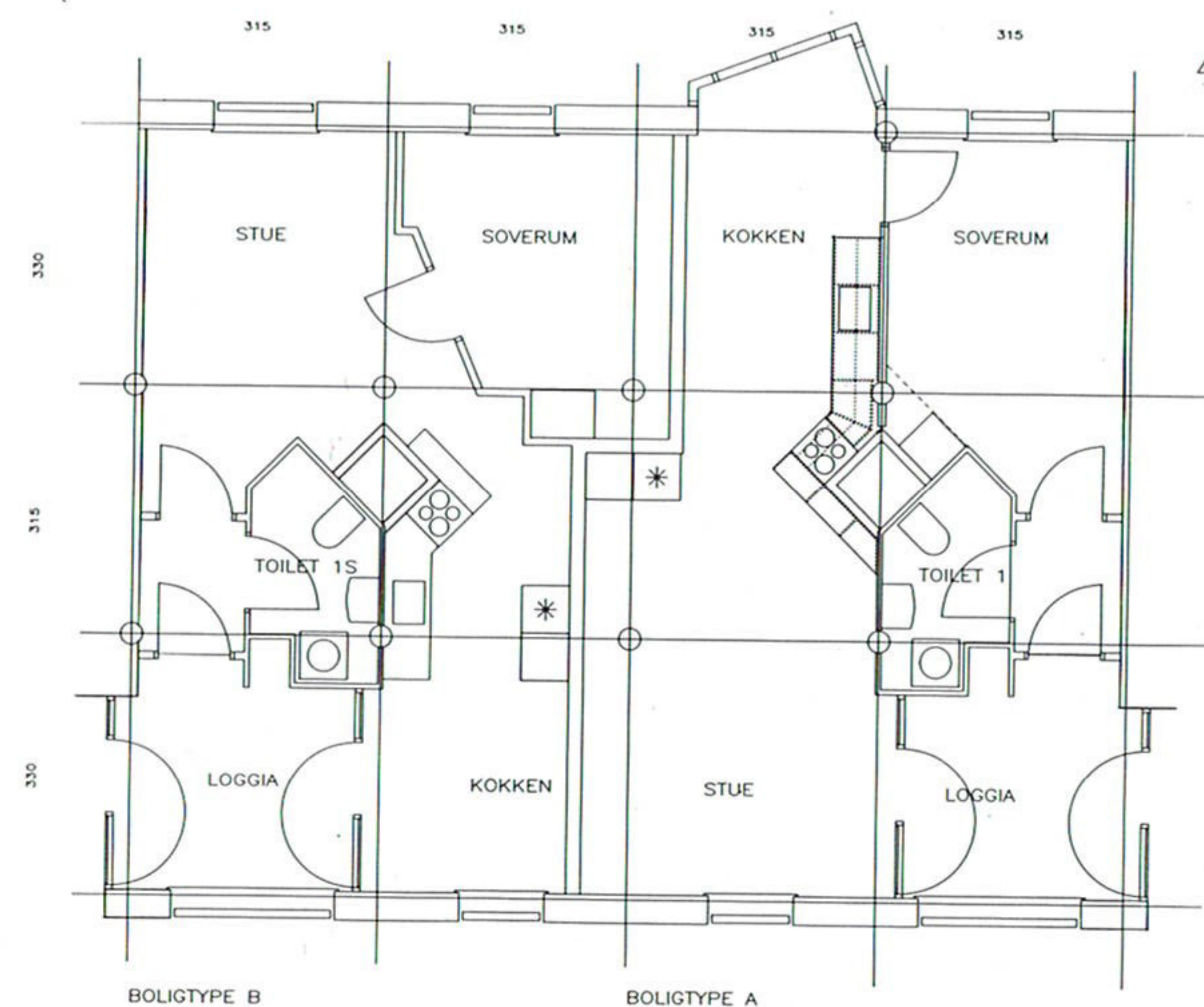
Eksempel på lejlighedsplaner.
